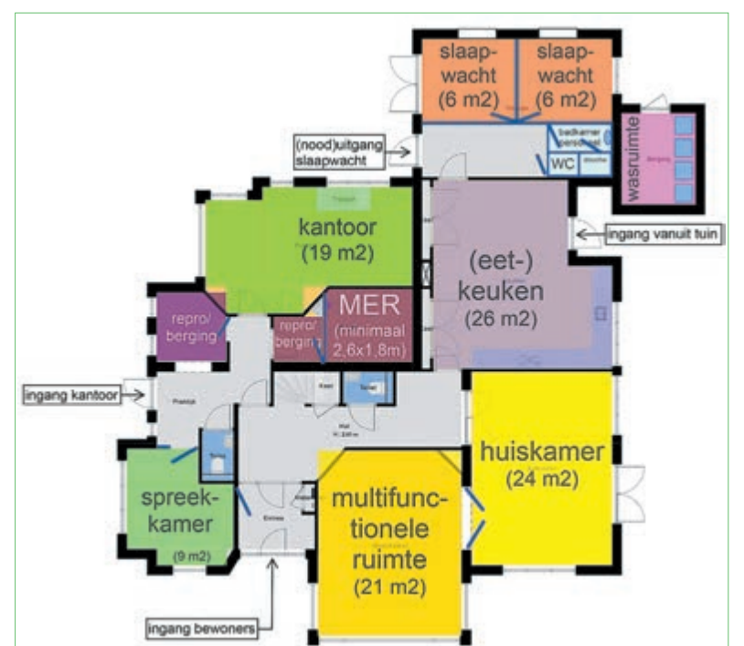
Deze bouwtekening geeft een indruk van de begane grond. Beeld aangeleverd.
